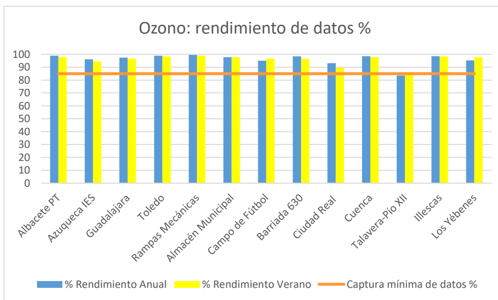
Figura 4.4.1.4. Calidad de los datos registrados para el Ozono
