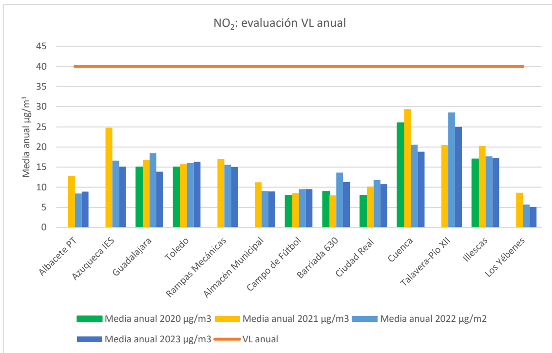
Figura 4.2.1.3. Evaluación del VL anual de NO 2 .
