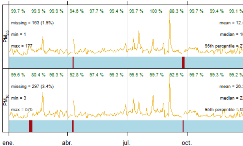
Estación de Cuenca - Evolución anual, 2023
