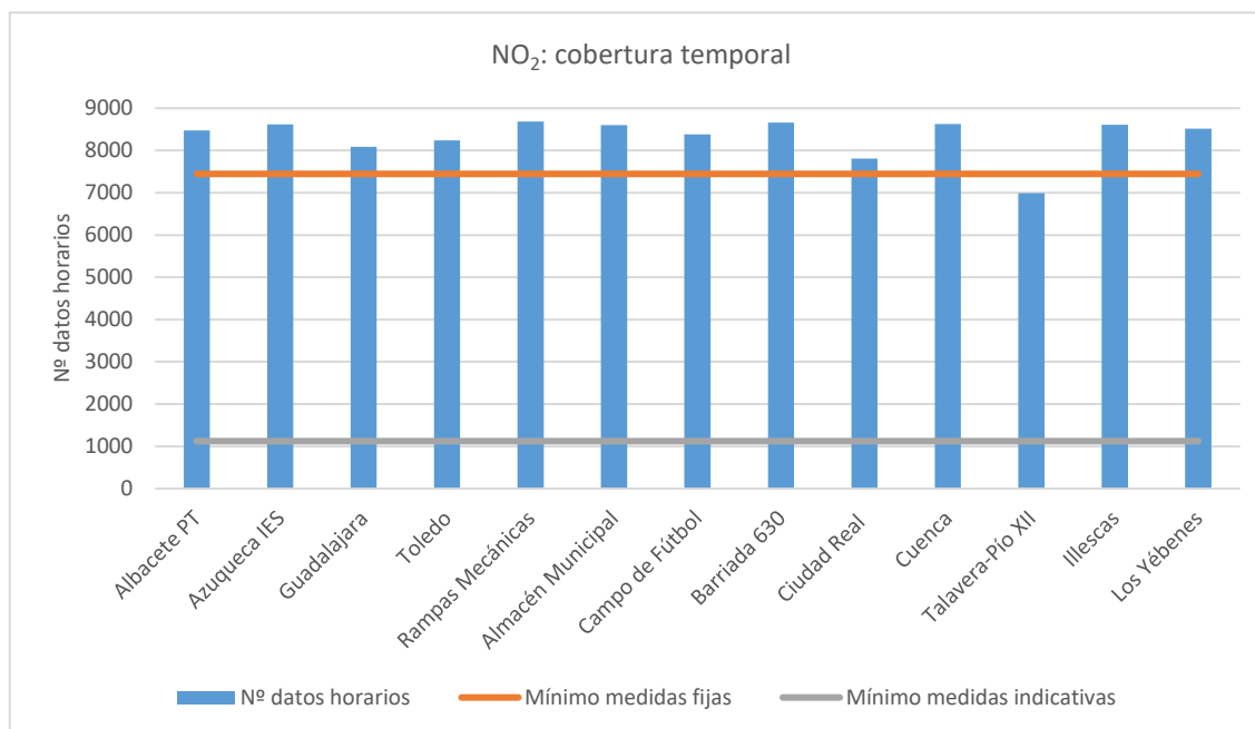
Figura 4.2.1.4. Calidad de los datos para NO 2 .
