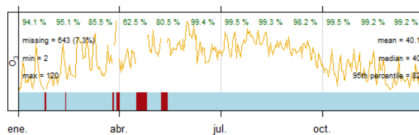
Estación de Talavera - Evolución anual, 2024
