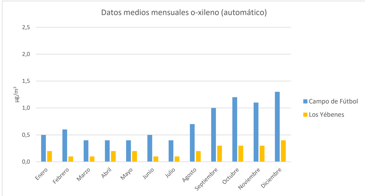
Figura 4.6.1.3.d. Evolución de las medias mensuales de o-xileno (datos automáticos).
