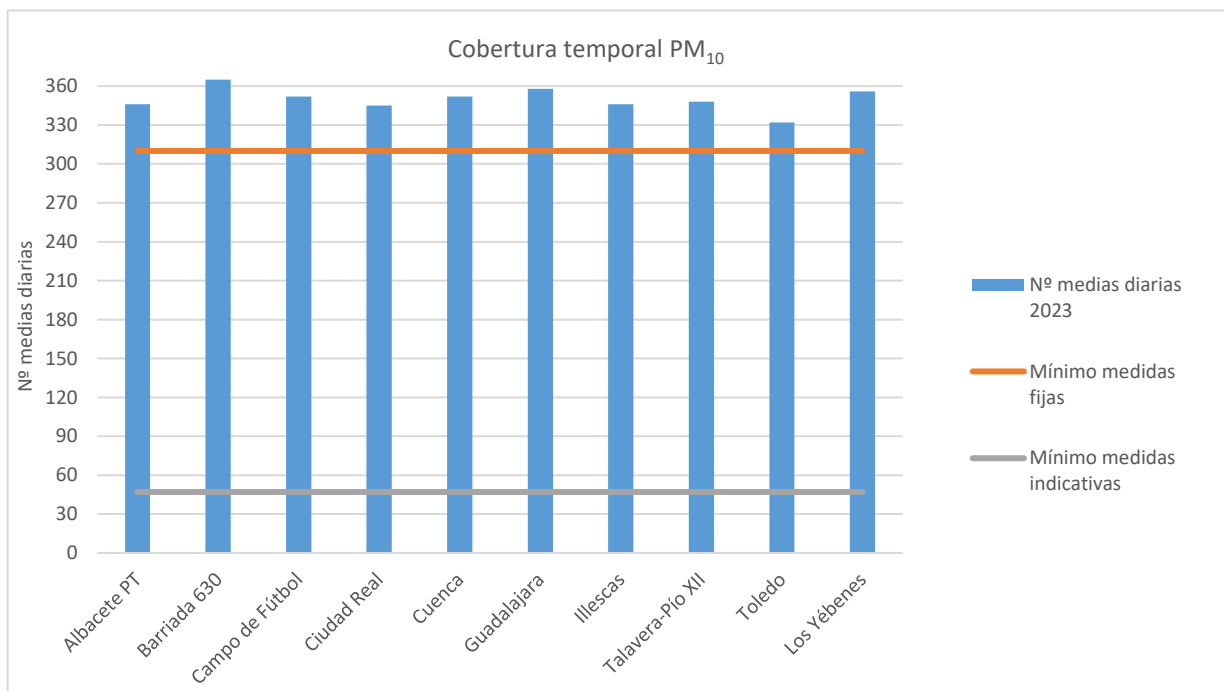
Figura 4.1.1.3. Calidad de datos-estaciones fijas para PM 10 : comparación número medias diarias con número de datos mínimos especificados en normativa.
