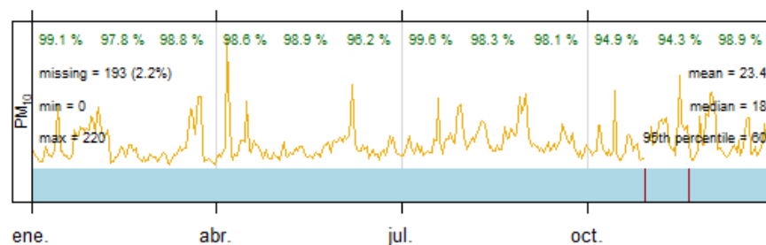
Estación de Barriada - Evolución anual, 2024
