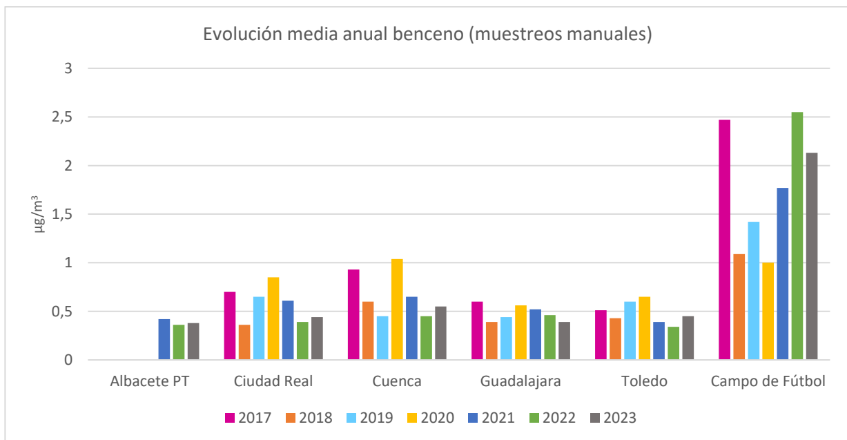
Figura 4.6.1.2. Evolución de las medias anuales de benceno 2017-2023 (muestréos manuales).
