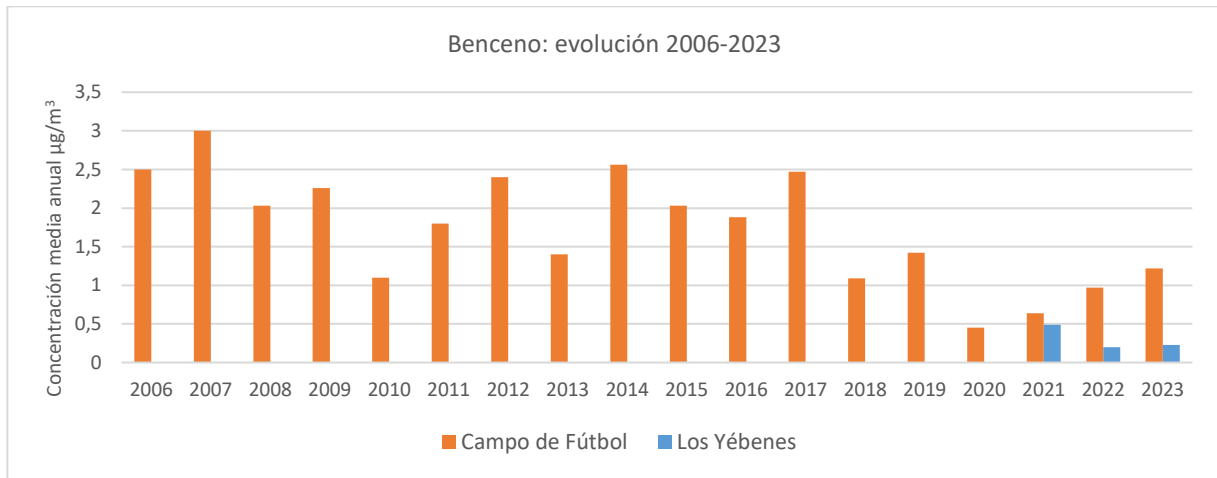
Figura 4.6.1.1. Evolución de las medias anuales de benceno 2006-2023 (analizadores actuales midiendo en continuo)
