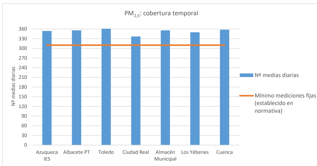
Figura 4.1.1.10. Cobertura temporal de datos de PM 2,5 .
