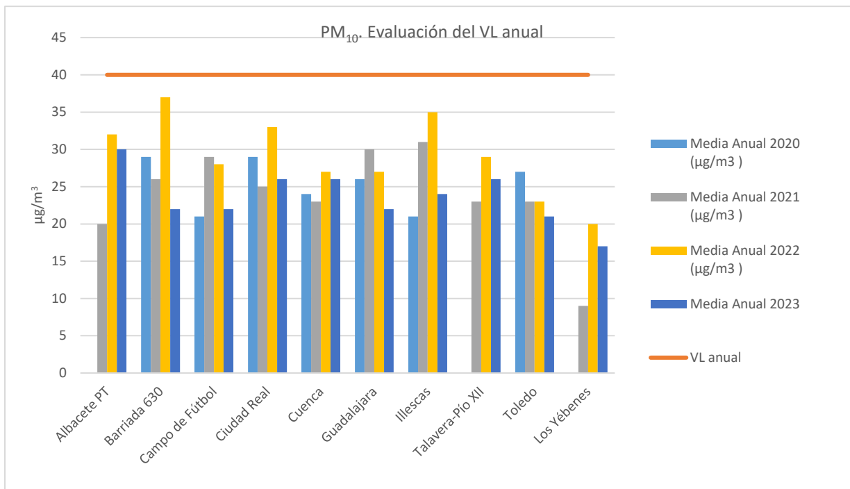
Figura 4.1.1.2. Evaluación del cumplimiento del VL anual de PM 10 .
