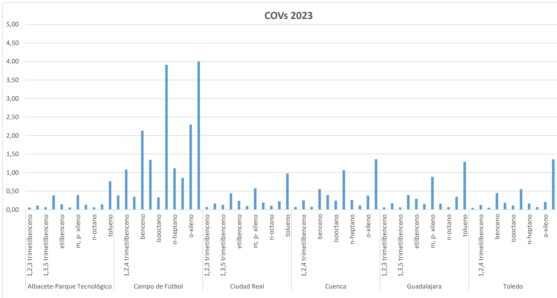
Figura 7.3.1 Datos COV's obtenidos de muestreos manuales 2023.
