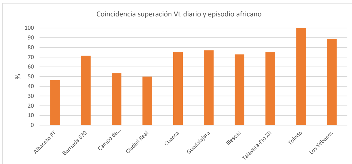
Figura 4.1.1.7. Días con superación del VL diario de PM 10 y con episodio de polvo africano. Datos descuentos: Ministerio para la Transición Ecológica y el Reto Demográfico (MITECO).
