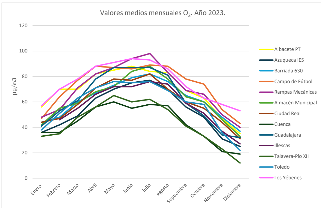
Figura 4.4.1.1. Evolución valores medios mensuales por estación.
