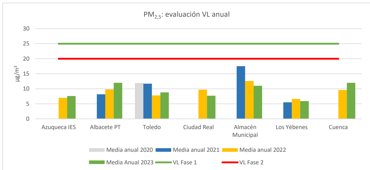
Figura 4.1.1.9. Evaluación VL anual de \text{PM}_{2,5} .
