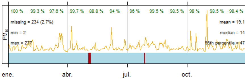
Estación de Guadalajara - Evolución anual, 2024
