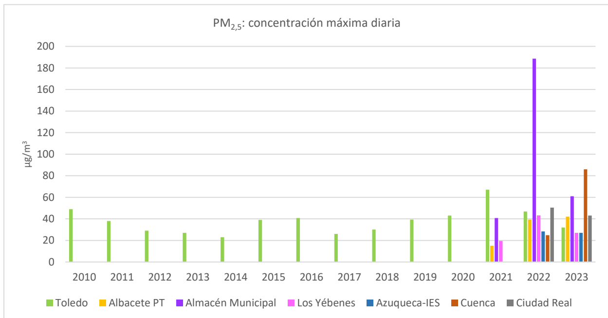
Figura 5.1.3.2. Evolución de la concentración máxima diaria PM 2,5 (puntos de muestreo activos en 2023).
