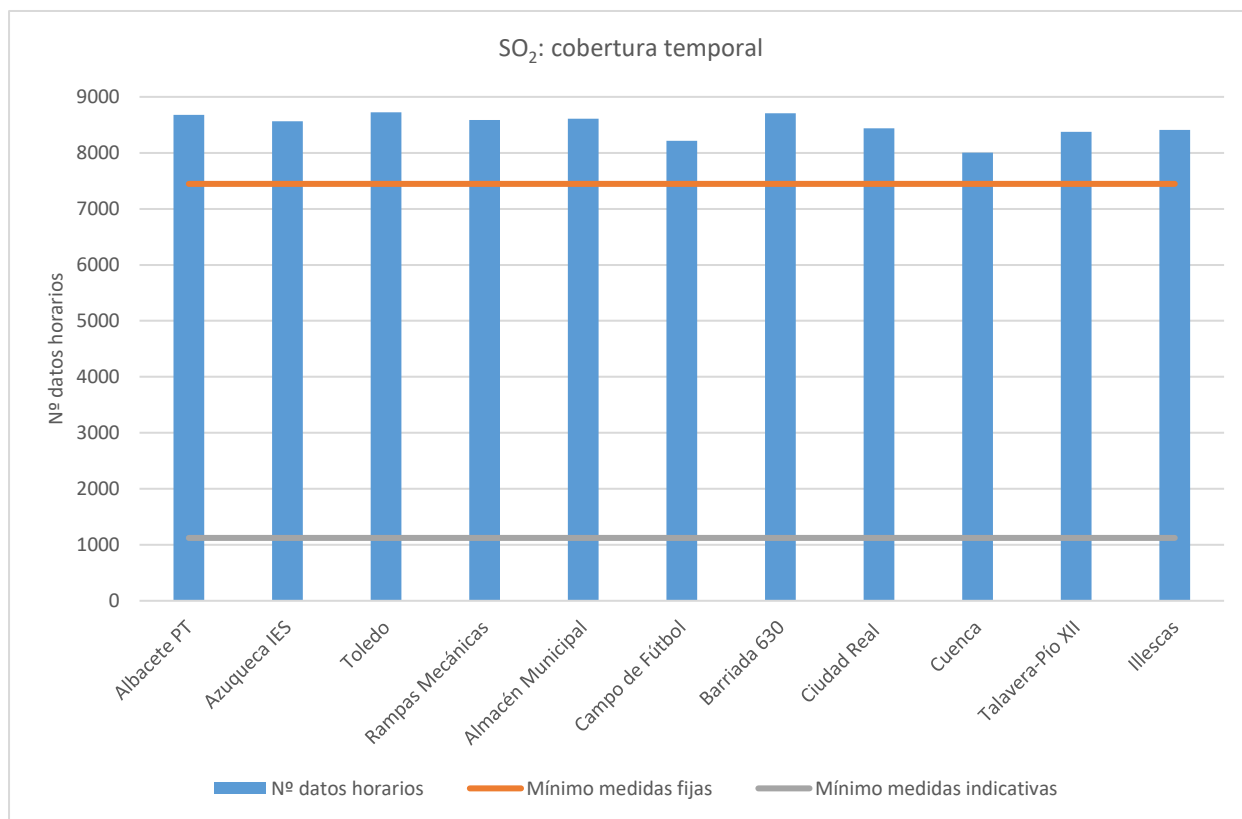
Figura 4.3.1.3. Calidad de datos registrados de SO 2 .
