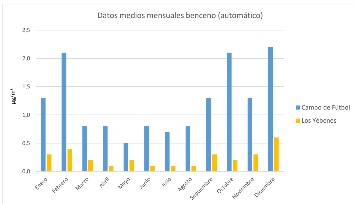
Figura 4.6.1.3.a. Evolución de las medias mensuales de benceno (datos automáticos).
