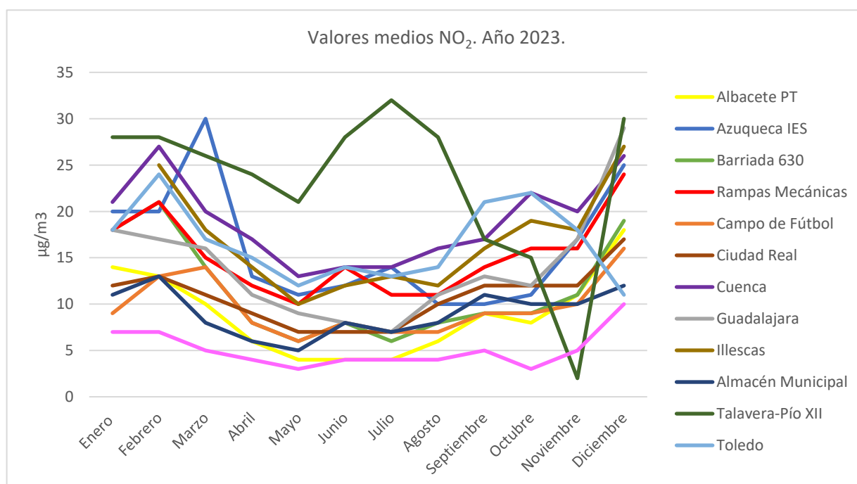
Figura 4.2.1.1. Evolución valores medios mensuales por estación.
