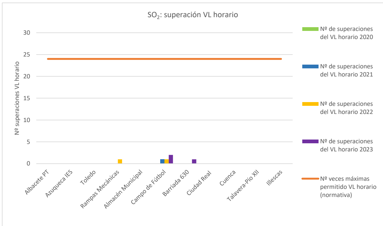
Figuras 4.3.1.2.b Evaluación cumplimiento valores límite para el SO 2 .
