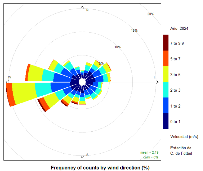
Figura 8.3.4. Rosa de los vientos; estación de Campo de Fútbol (Puertollano).
