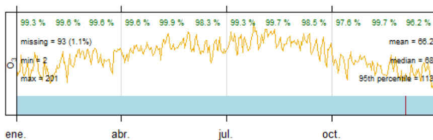
Estación de Rampas Mecánicas - Evolución anual, 2024
