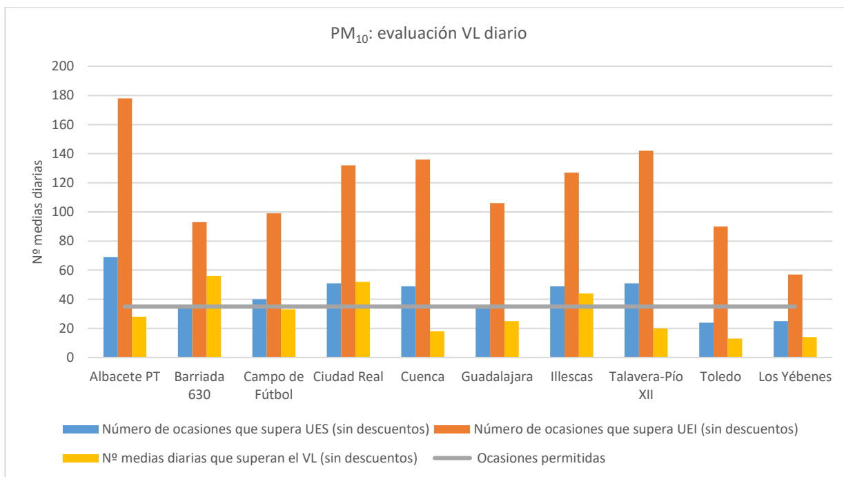
Figura 5.1.1.1. Evaluación del VL diario y umbrales de \text{PM}_{10} , sin aplicar descuentos por intrusiones de polvo africano
