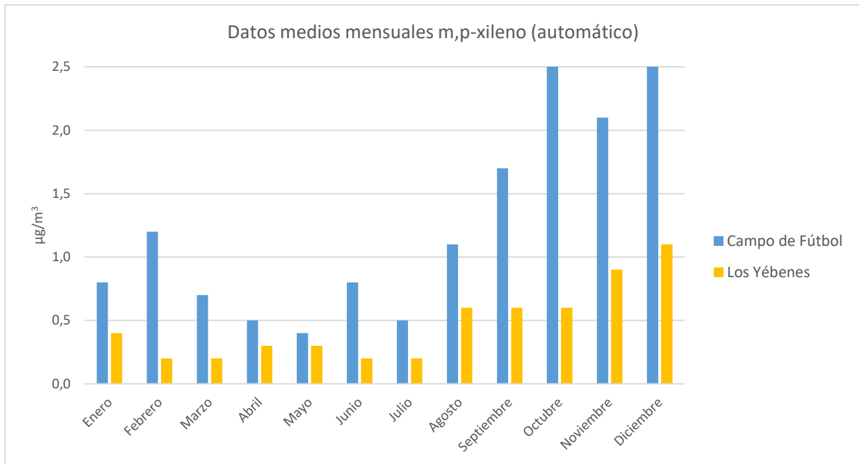
Figura 4.6.1.3.c. Evolución de las medias mensuales de m,p-xileno (datos automáticos).
