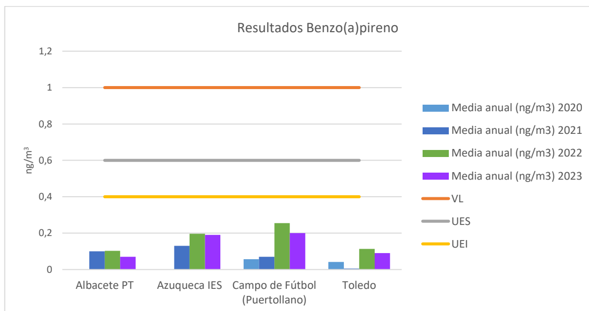
Figura 7.2.1. Resultados benzo(a)pireno 2023 y comparativa con 2020, 2021 y 2022.
