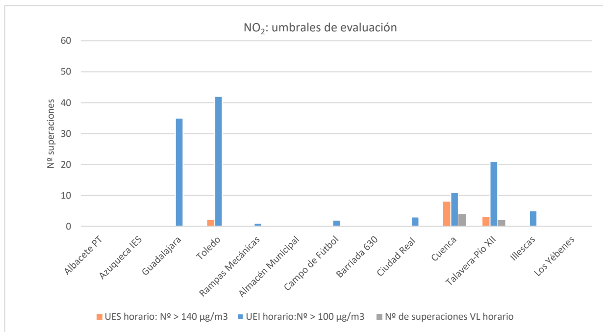
Figura 5.2.2.1. Umbrales de evaluación para el NO 2 .
