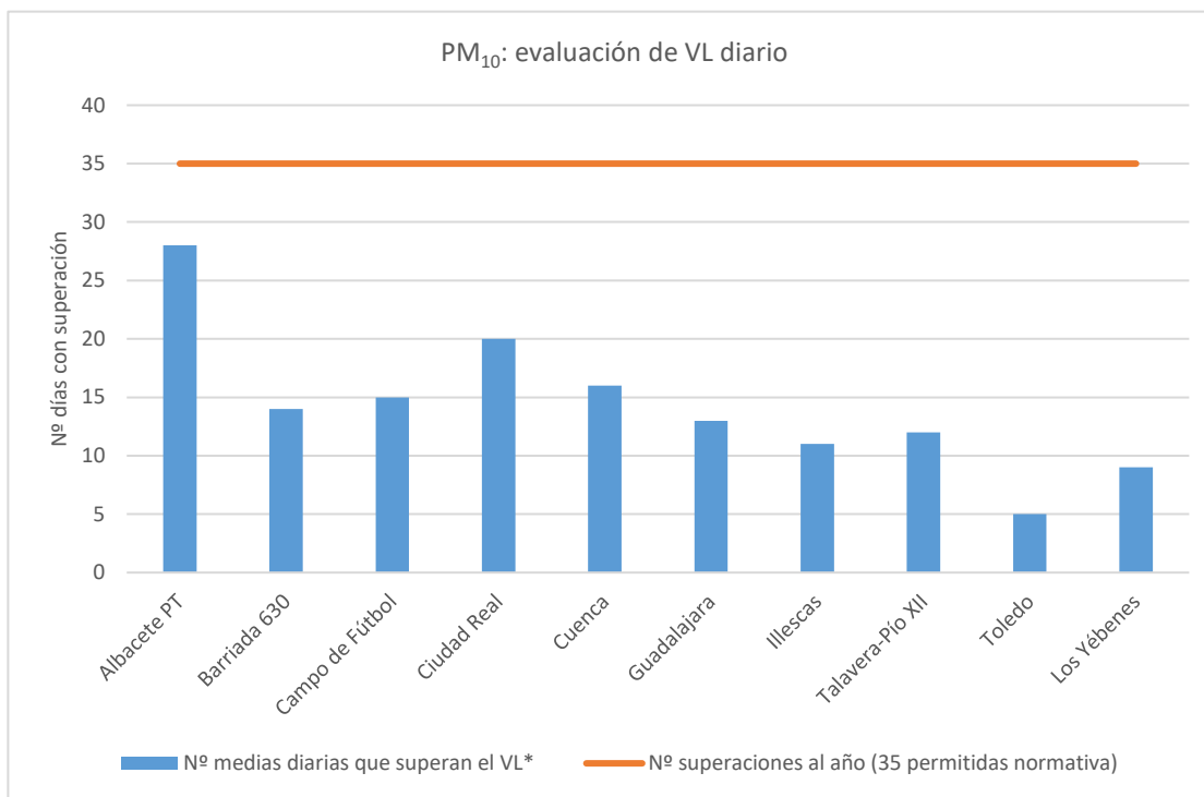
Figura 4.1.1.4. Cumplimiento del VL diario de PM 10 .
