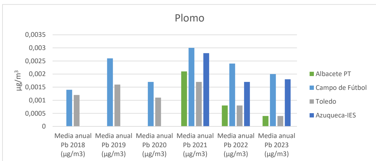
Figura 7.1.1 Resultados muestreos de metales 2018, 2019, 2020, 2021,2022 y 2023
