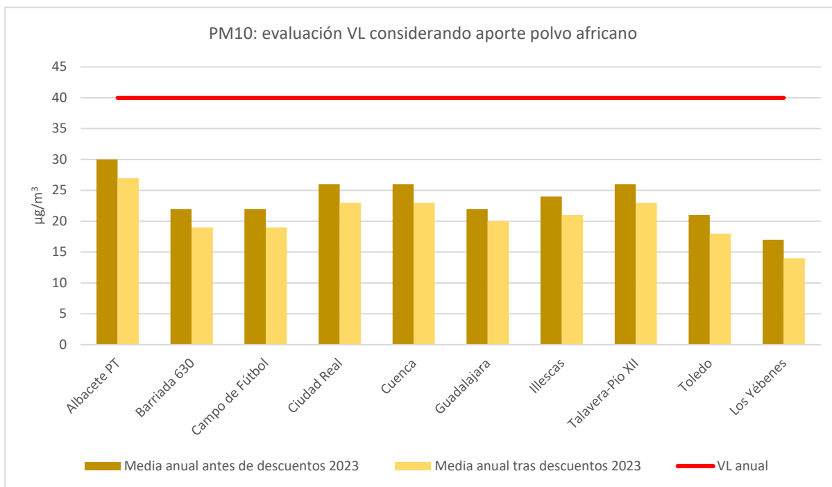
Figura 4.1.1.5. Evaluación cumplimiento VL anual para PM 10 antes y tras descuentos.
