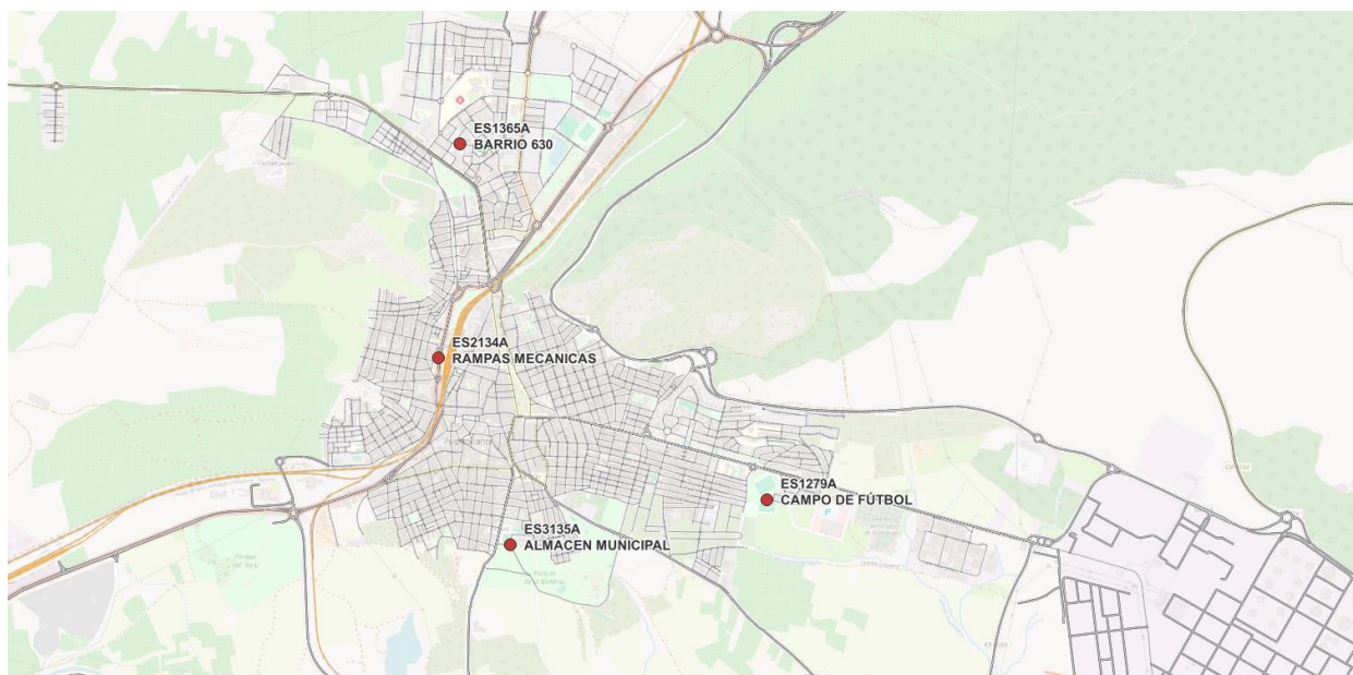
Figura 2.1.2. Estaciones públicas de la Red de Control y Vigilancia de la Calidad del Aire de Castilla-La Mancha en Puertollano -Año 2023
