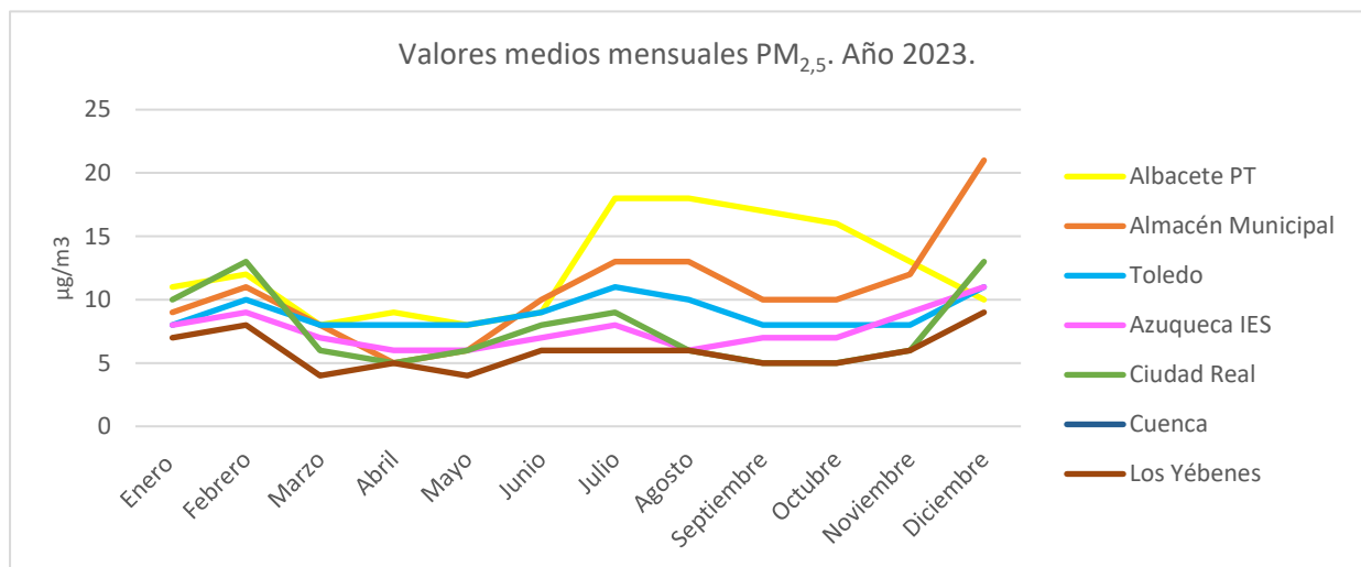
Figura 4.1.1.8. Evolución valores medios mensuales \text{PM}_{2,5} por estación.
