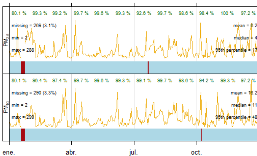
Estación de Los Yébenes - Evolución anual, 2024
