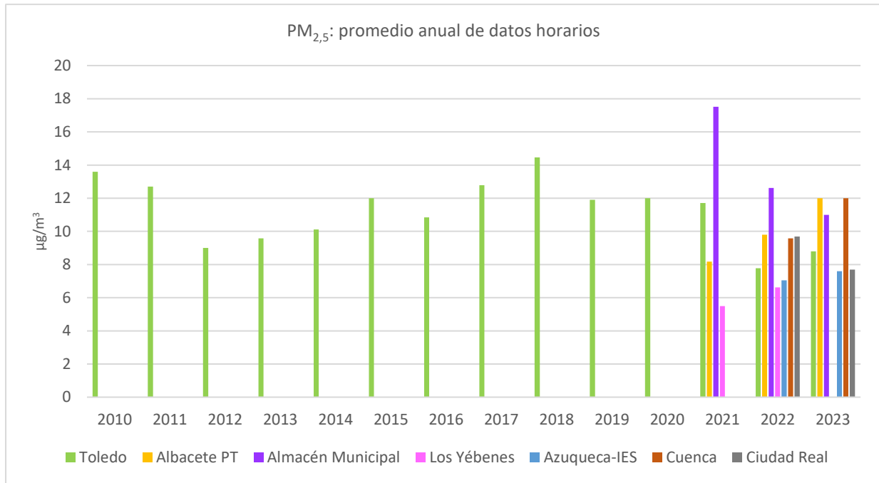
Figura 5.1.3.1. Evolución del promedio anual de datos horarios PM 2,5 (puntos de muestreo activos en 2023).
