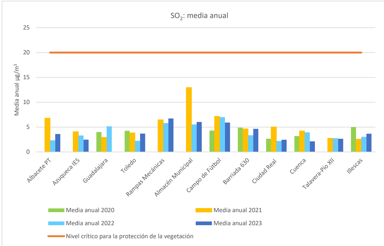
Figuras 4.3.1.2.a Evaluación cumplimiento valores límite para el SO 2
