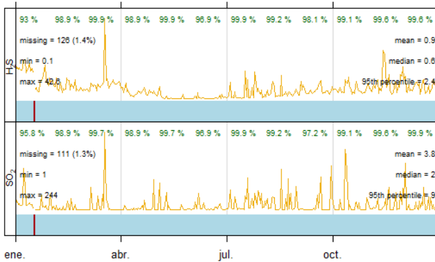
Estación de Barriada - Evolución anual, 2024
