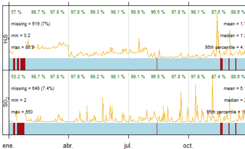
Estación de Campo de Fútbol - Evolución anual, 2024
