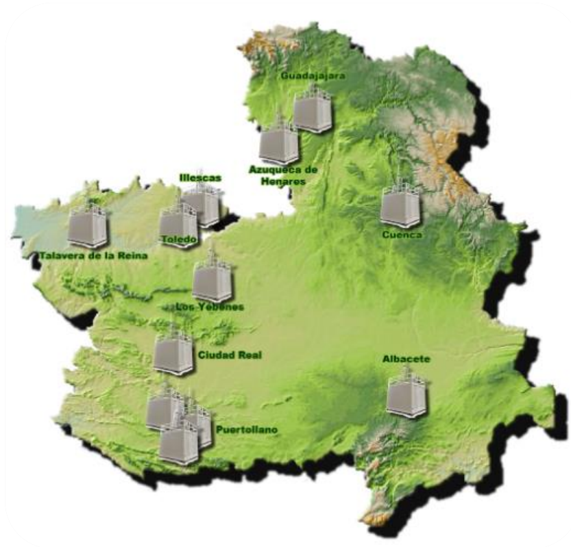
Figura 2.1.1. Estaciones públicas de la Red de Control y Vigilancia de la Calidad del Aire de Castilla-La Mancha. Año 2023.
