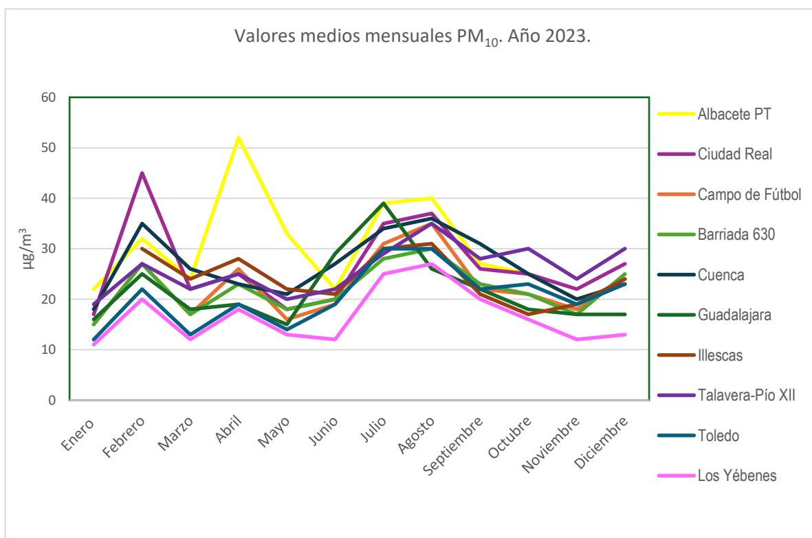
Figura 4.1.1.1. Evolución valores medios mensuales por estación
