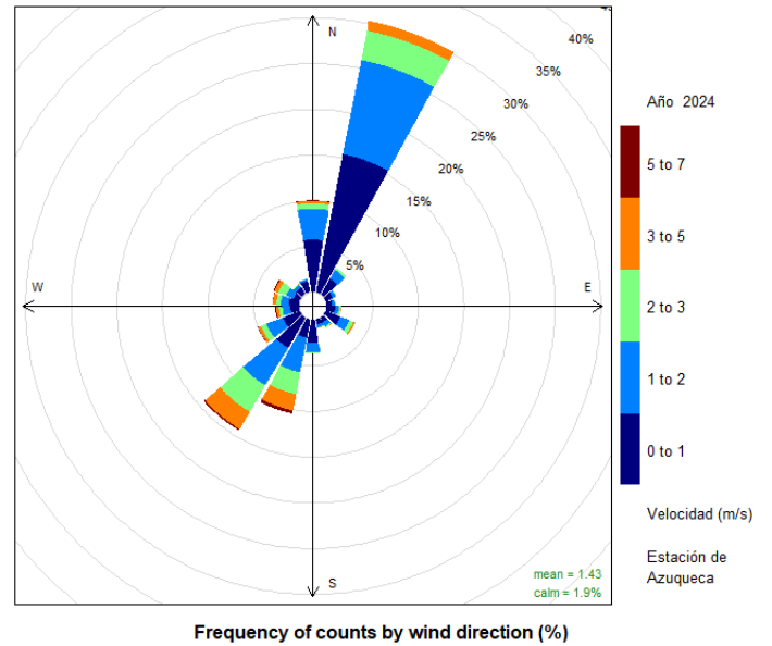
Figura 8.3.2. Rosa de los vientos; estación de Azuqueca IES.
