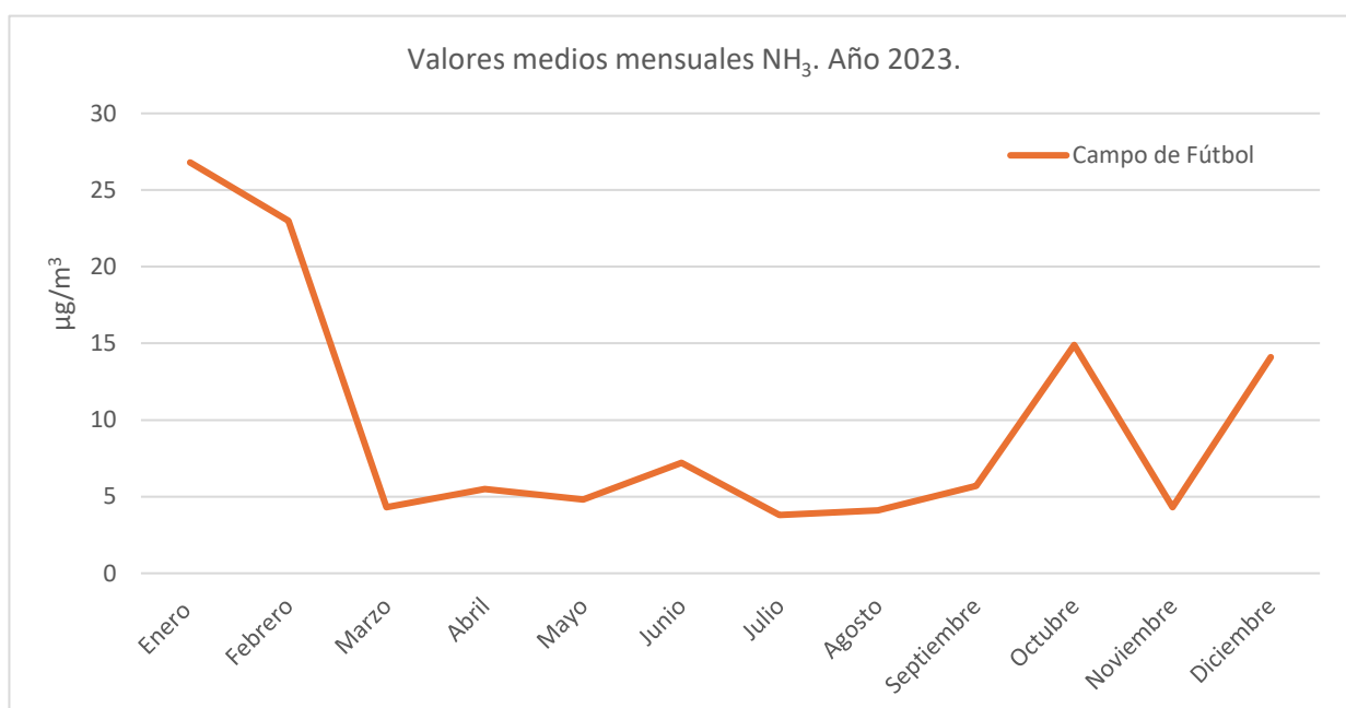
Gráfico 4.7.1.1. Evolución de las medias mensuales para amoniaco. Año 2023.
