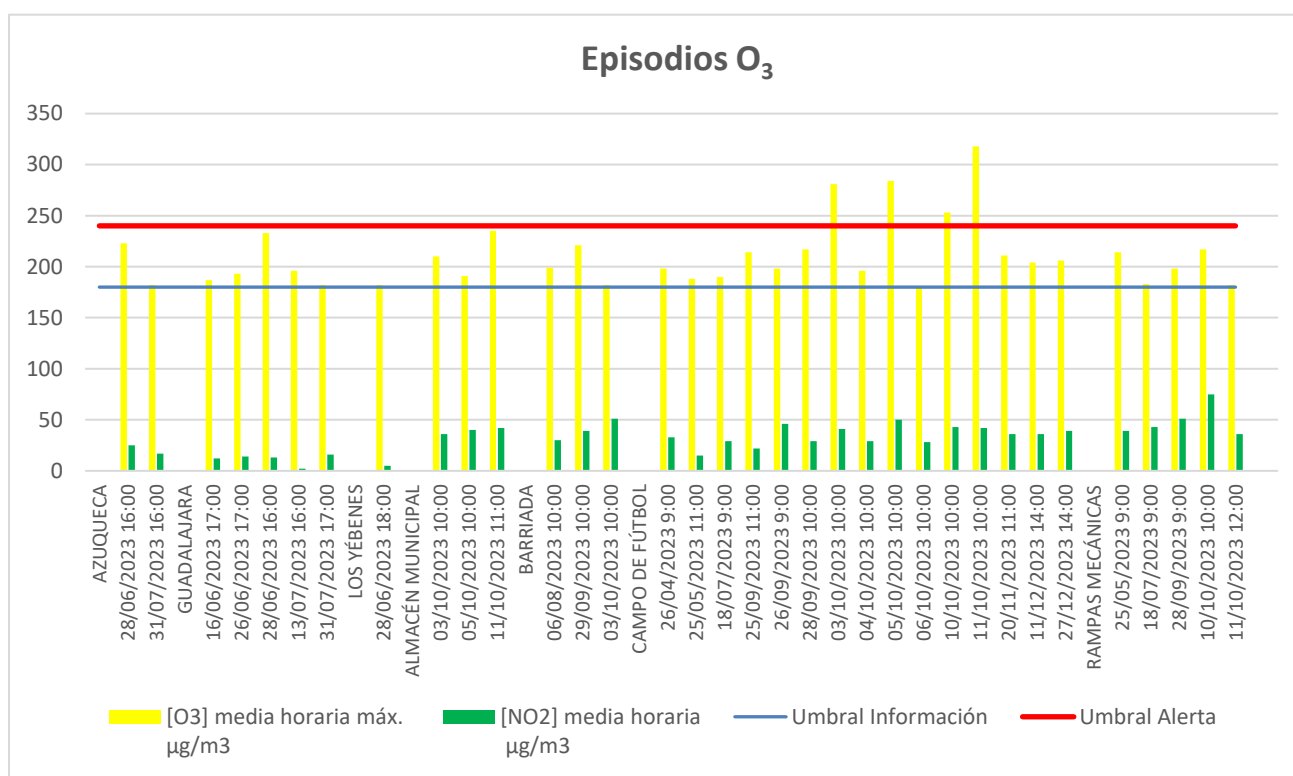
Figura 5.4.1.1 Episodios ozono registrados en el año 2023 (Hora UTC).
