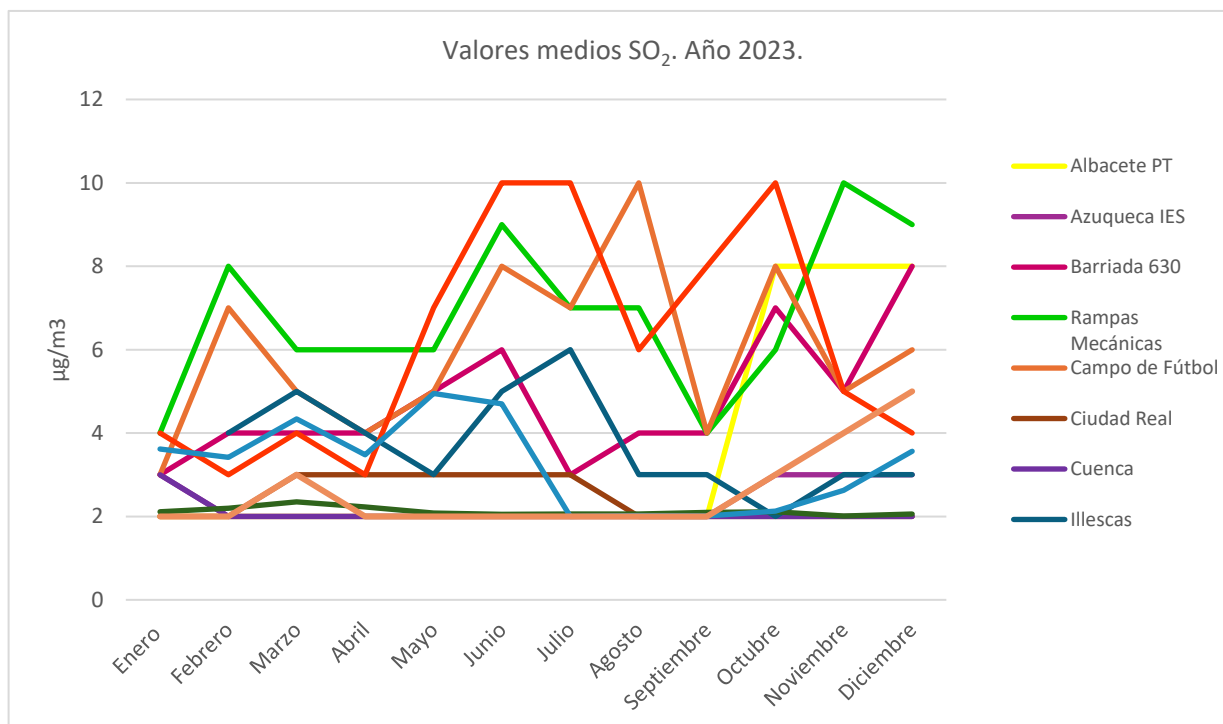
Figura 4.3.1.1. Evolución valores medios mensuales por estación.
