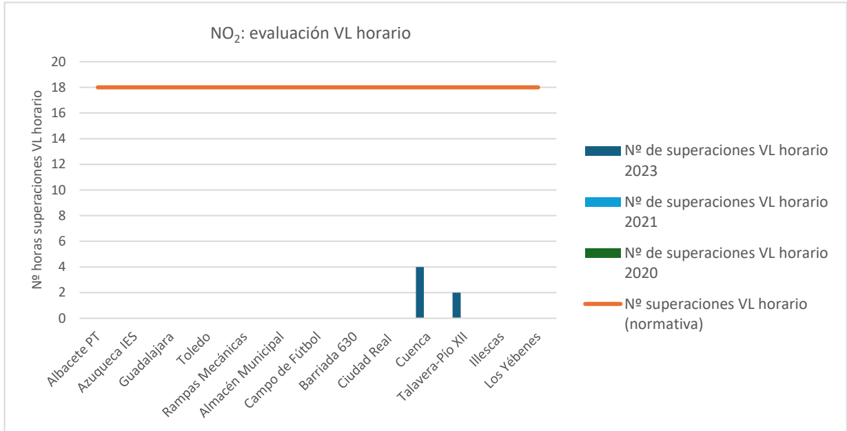
Figura 4.2.1.2. Evaluación del VL horario de NO 2 .
