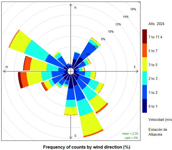
Figura 8.3.1. Rosa de los vientos; estación de Albacete PT.
