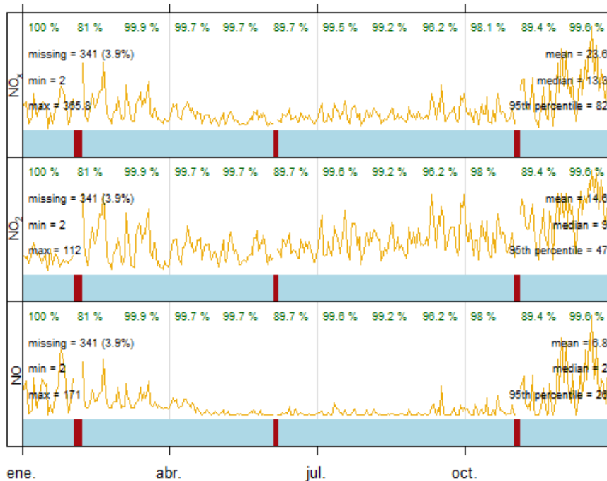
Estación de Toledo - Evolución anual, 2024
