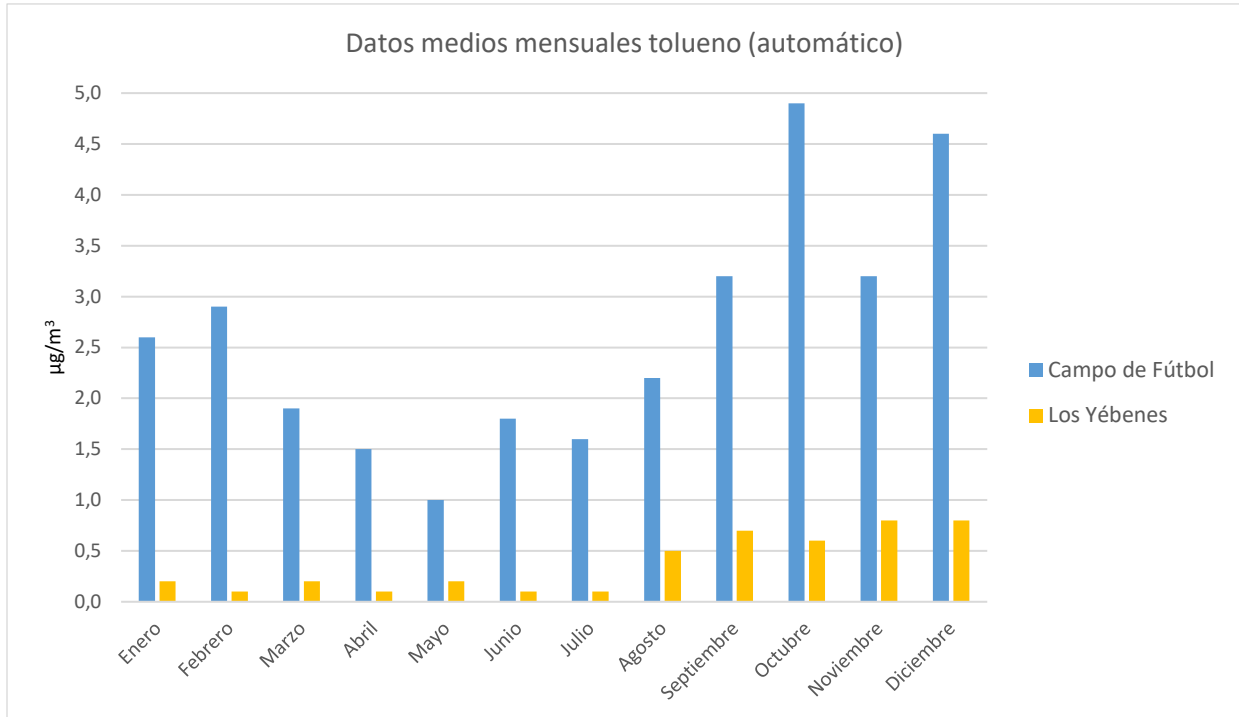
Figura 4.6.1.3.b. Evolución de las medias mensuales de tolueno (datos automáticos).
