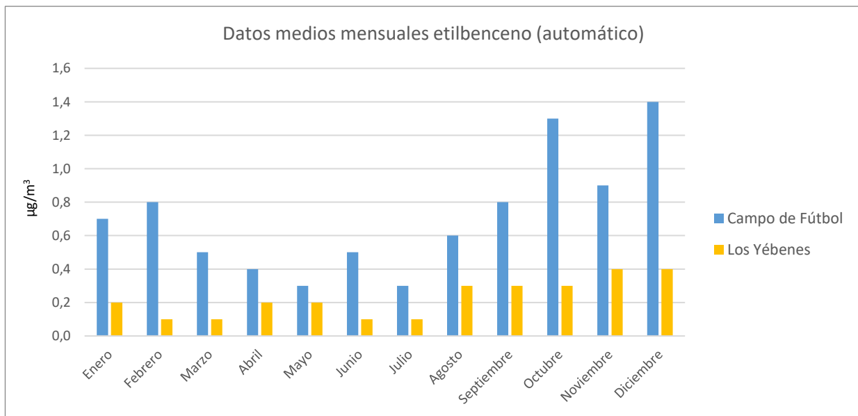
Figura 4.6.1.3.e. Evolución de las medias mensuales de etilbenceno (datos automáticos).
