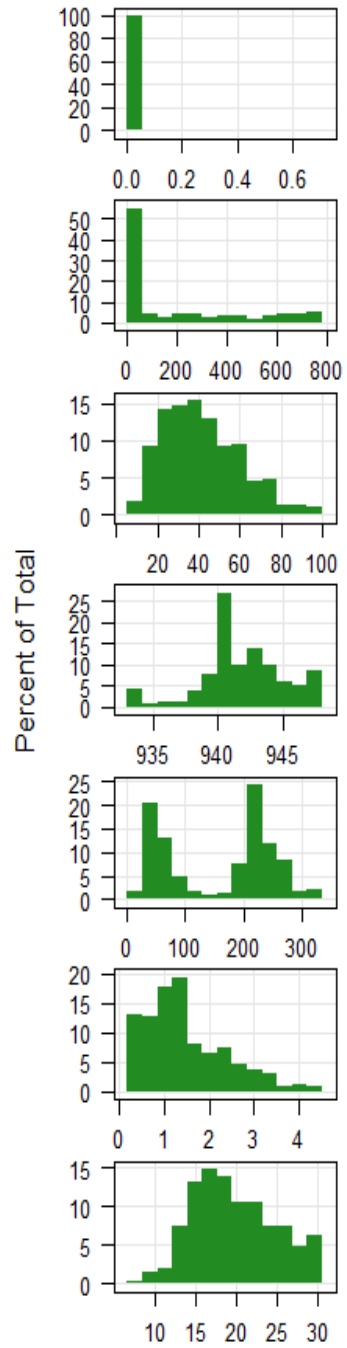
Histogramas
