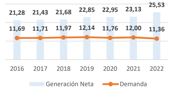
Evolución de la Generación y la Demanda de Energía en Castilla-La Mancha (TWh)
